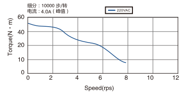
力矩曲线
